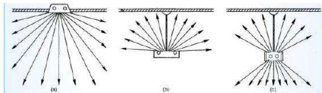
Рис. 203. Світильники:
