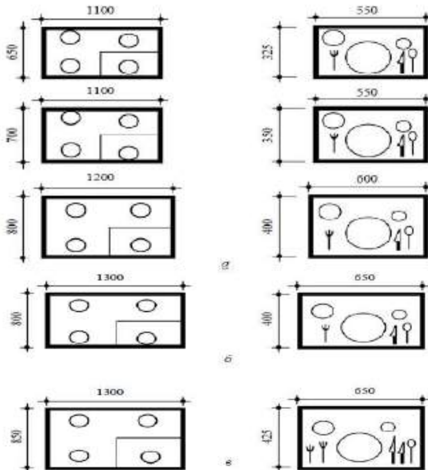
Рис. 190. Параметри обідньої площини за різних розмірів сервірувального посадочного місця: a – побутова; б – для їдалень і кафе; в – для ресторанів
