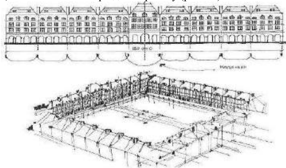
Рис. 20. Симетрія переносу
