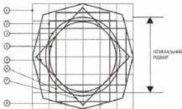
Рис. 264. Конфігуратор
