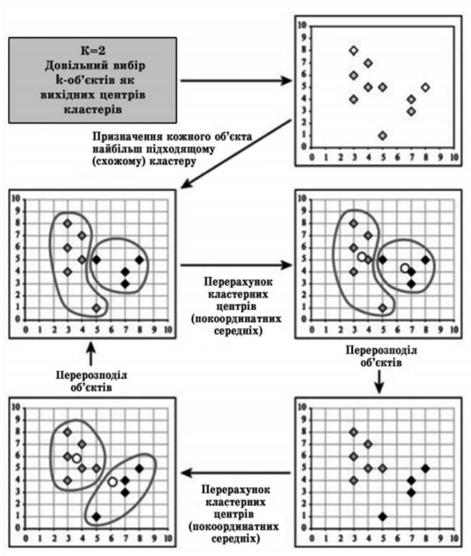
Рис. 3.14. Приклад роботи алгоритму k-середніх для k = 2
