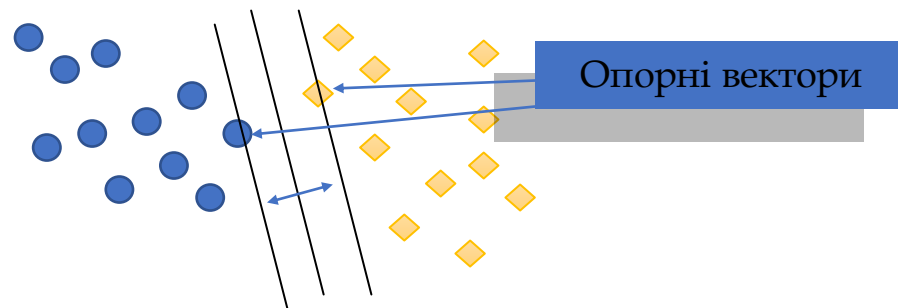
Рис. 3.5. До визначення опорних векторів
