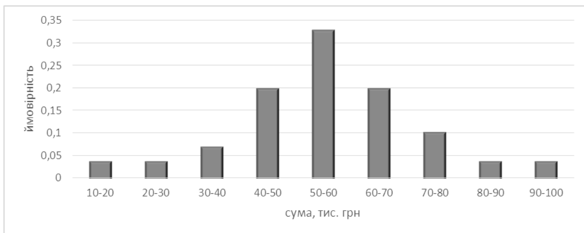
Рис. 2.32. Нормована гістограма
