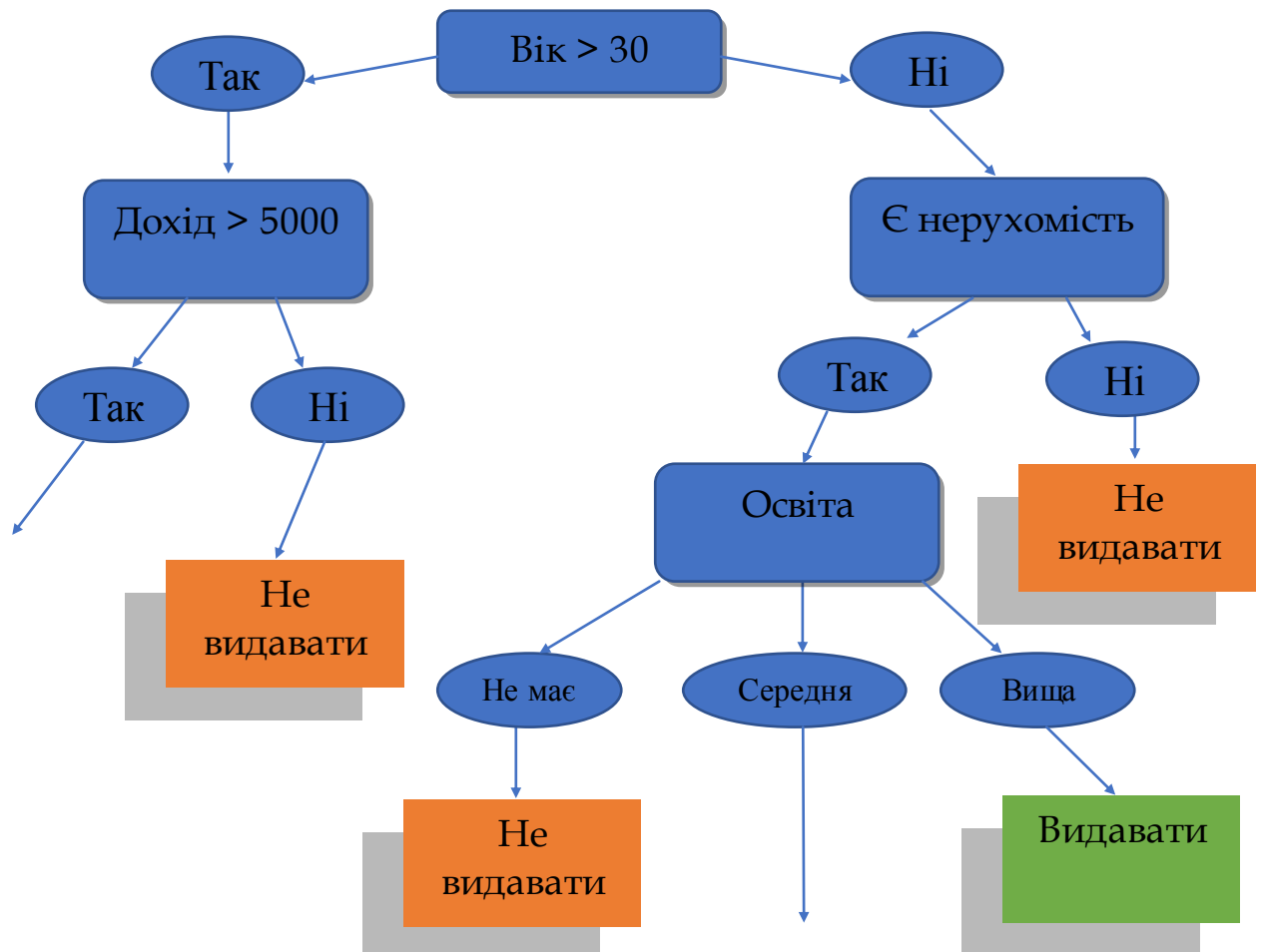
Рис. 3.3. Дерево класифікації
