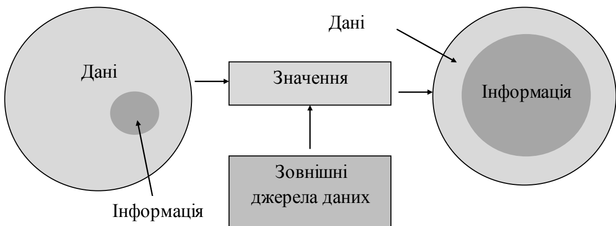
Рис. 2.24. Збагачення даних
