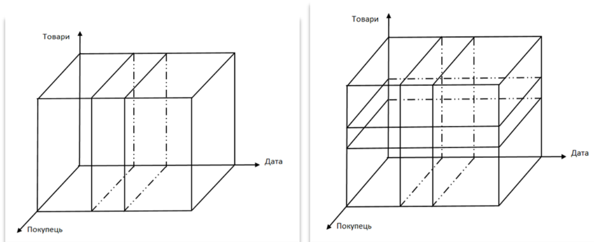
Рис. 2.7. Перетини гіперкуба
