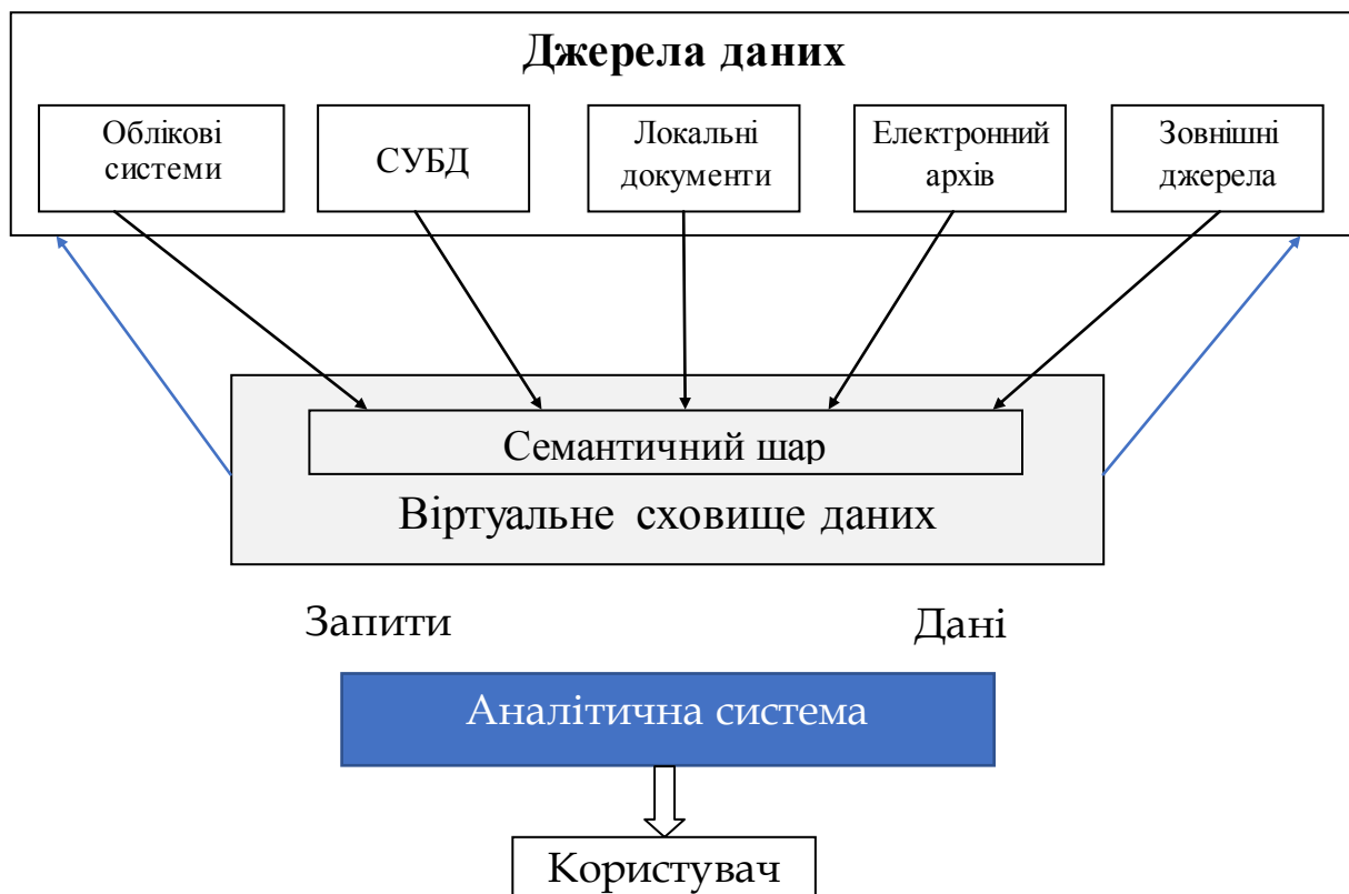
Рис. 2.13. Віртуальне СД
