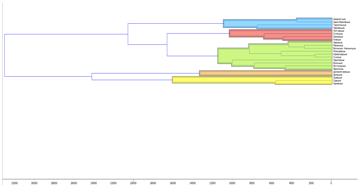
Рис. 2.47. Приклад дендрограми
