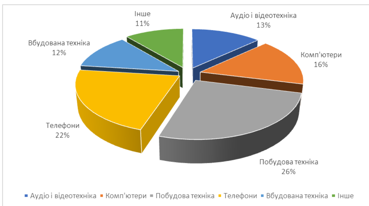
Рис. 2.29. Кругова діаграма
