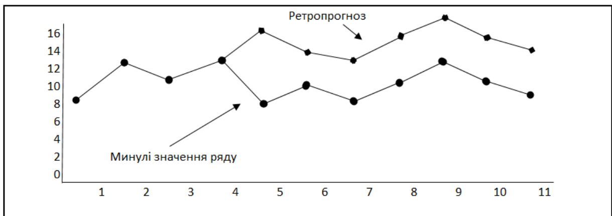
Рис. 2.43. Діаграма ретропрогнозу
