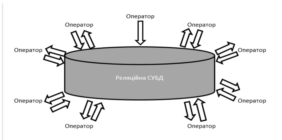
Рис. 2.2. OLTP-система
