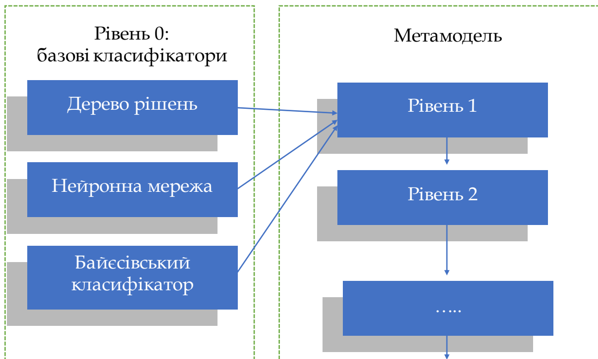
Рис. 3.15. Стекінг
