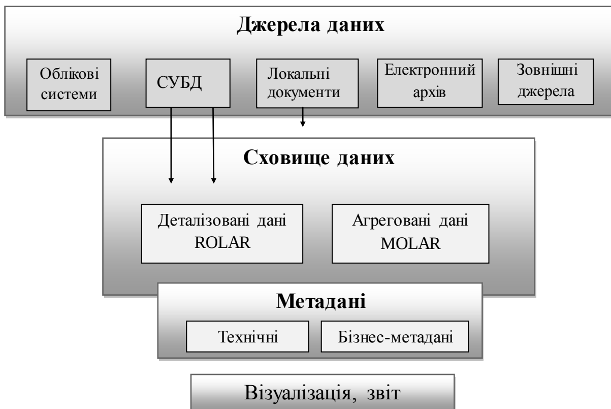
Рис. 2.10. Гібридне СД
