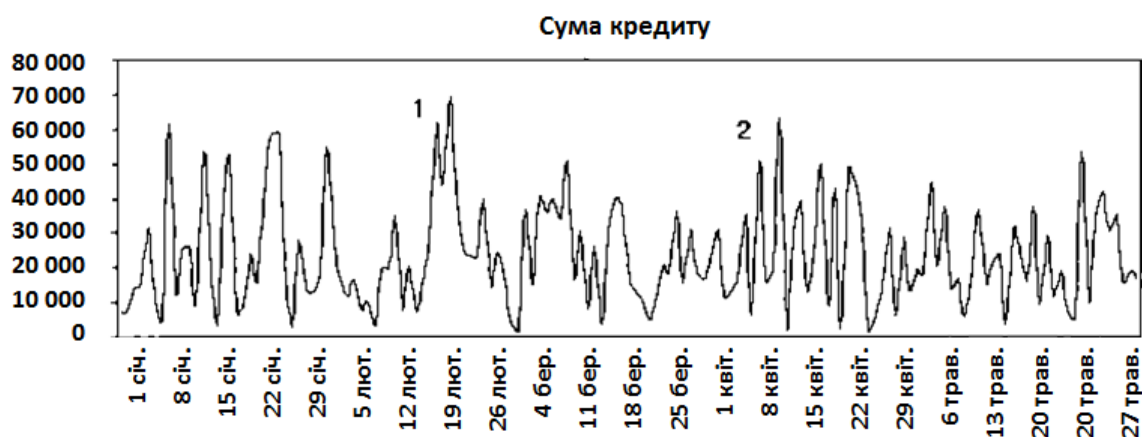
Рис. 2.54. Ряд даних
