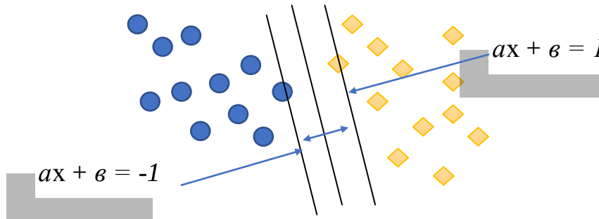
Рис. 3.6. Лінійний SVM
