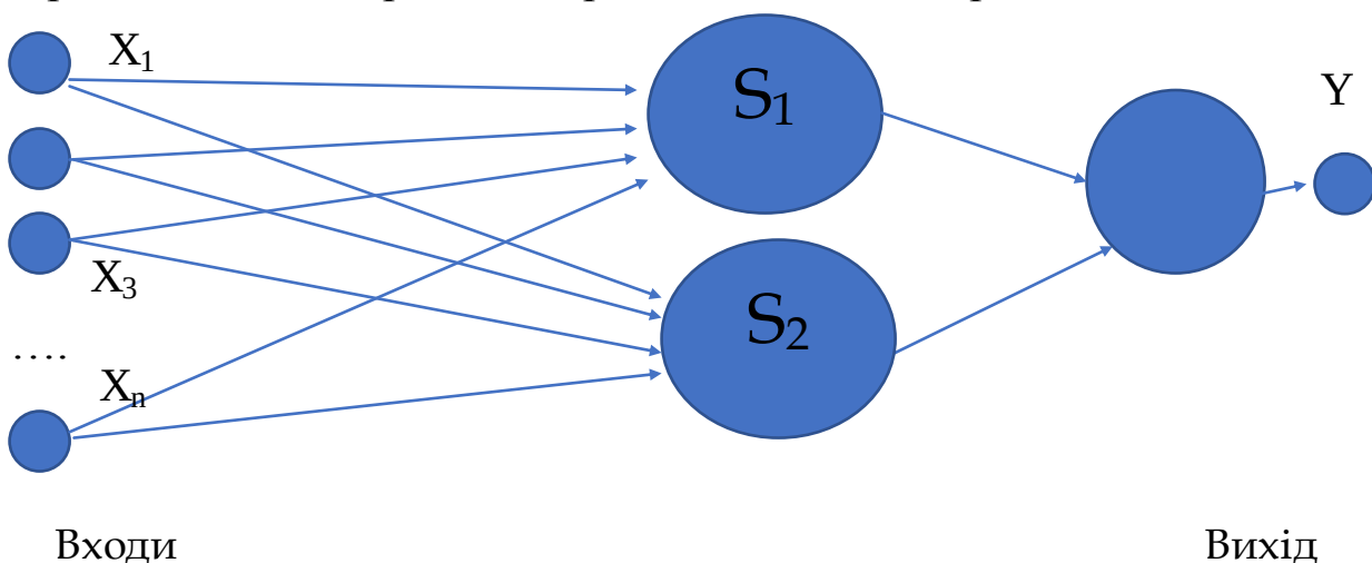
Рис. 3.9. Одношаровий персептрон
