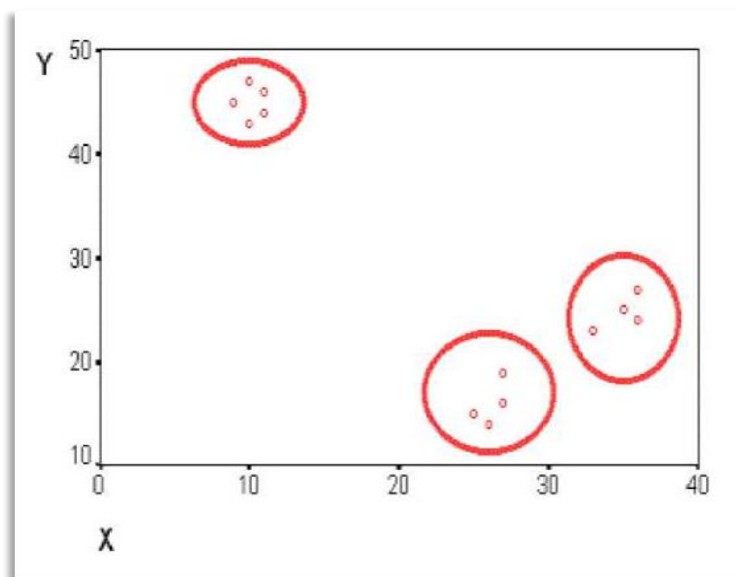
Рис. 3.11. Діаграма розсіювання
