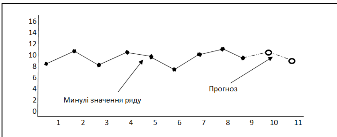
Рис. 2.42. Діаграма прогнозу
