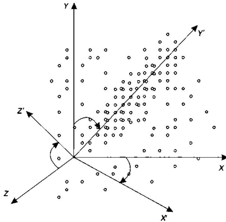
Рис. 2.57. Метод головних компонент
