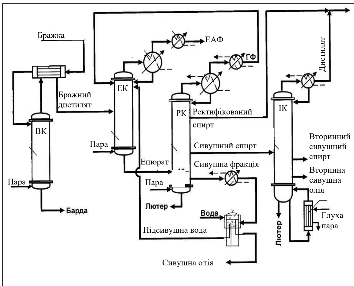
Рис. 8.6. Схема брагоректифікаційної установки:
