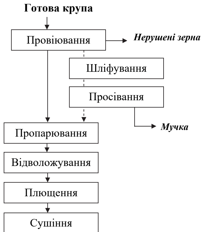
Рис. 3.18. Загальна схема виробництва зернових пластівців
