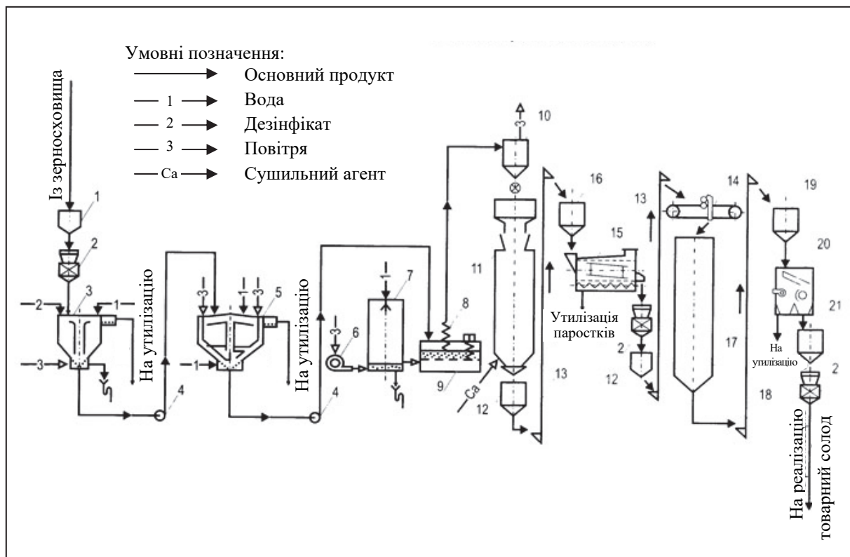
Рис. 7.4. Апаратурно-технологічна схема виробництва солоду:
