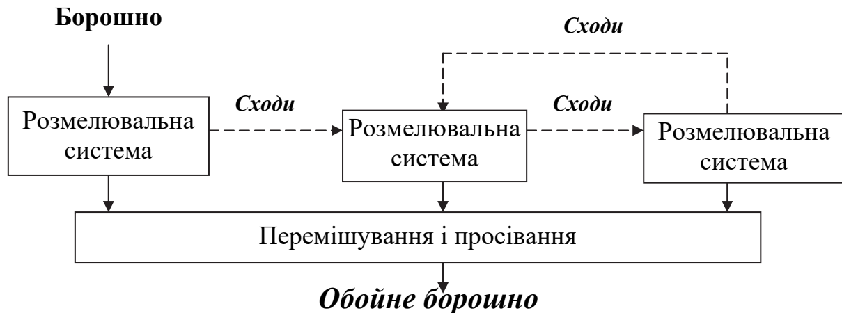
Рис. 3.10. Схема обдирного помелу
