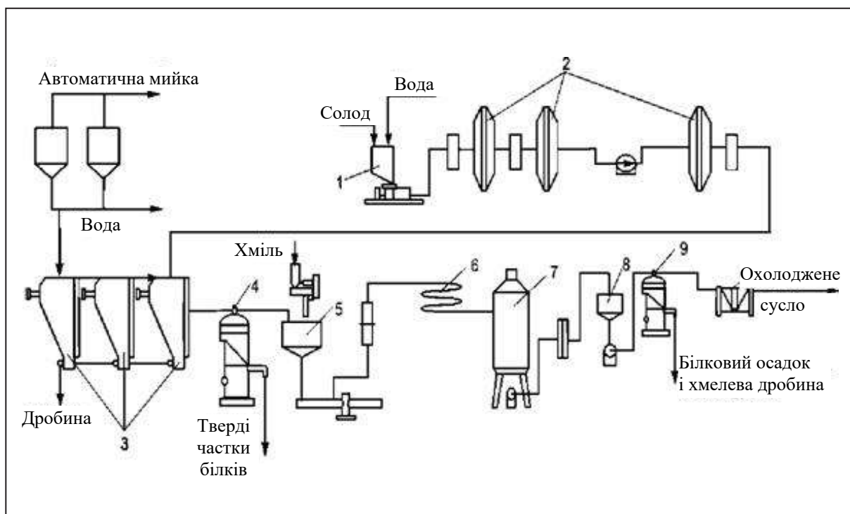
Рис. 7.8. Установа для безперервного виробництва сусла: 1 – заторний апарат; 2 – теплообмінники; 3 – промивник дробини; 4, 9 – сепаратори; 5 – змішувач; 6 – теплообмінник; 7 – вакуум-апарат; 8 – збірник сусла; 10 – холодильник
