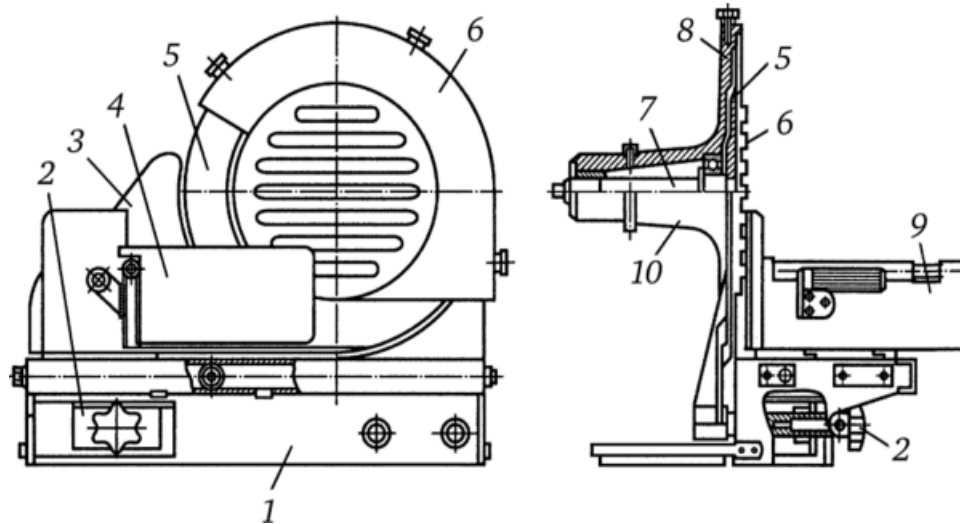
Рис. 42 – Схема механізму для нарізання гастрономічних товарів та хліба MKW-250:
