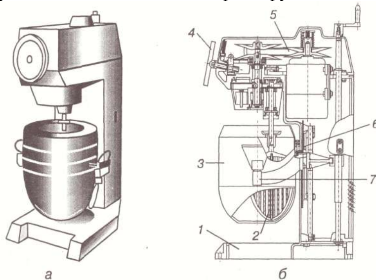
Рис. 54 – Машина збивальна MB-35M:
