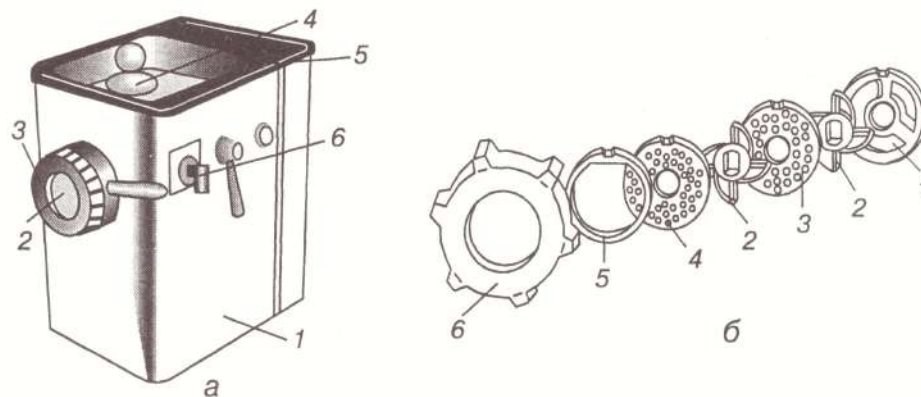
Рис. 29 – Принципова схема конструкції м'ясорубки:
