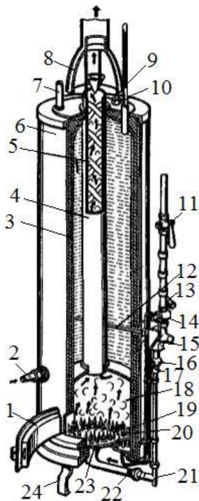
Рис. 99 – Водонагрівач типу АГВ-80:
