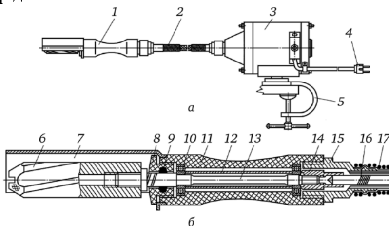
Рис. 38 – Схема пристрою для обчищення риби від луски:
