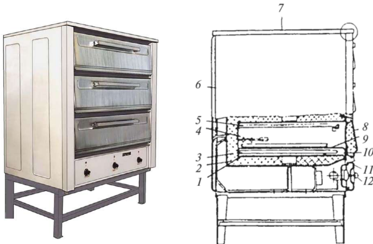
Рис. 80 – Шафа пекарська ШПЕСМ-3:
