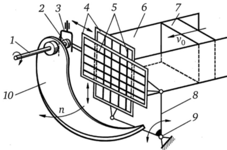
Рис. 35 – Принципова схема ріжучого вузла шпигорізки:
