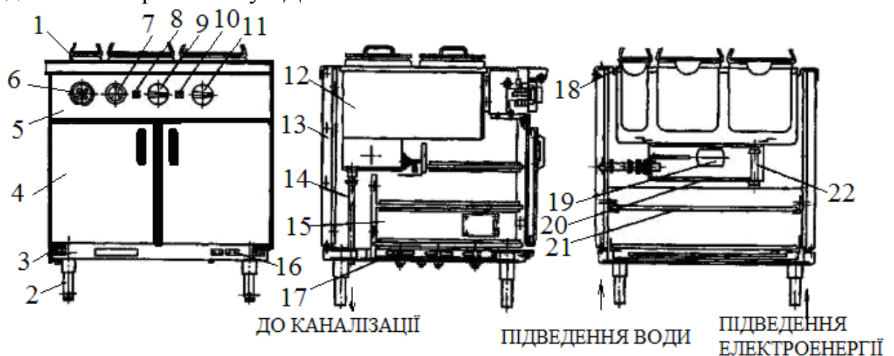
Рис. 101 – Марміт стаціонарний електричний секційний модульований МЕСЕМ-50:
