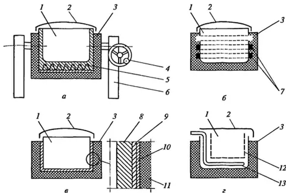
Рис. 54 – Принципові схеми електричних котлів з безпосереднім обігрівом стінки варильного посуду:
