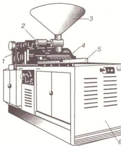
Рис. 51 – Машина МТВ для відсаджування заготівок із тіста:
