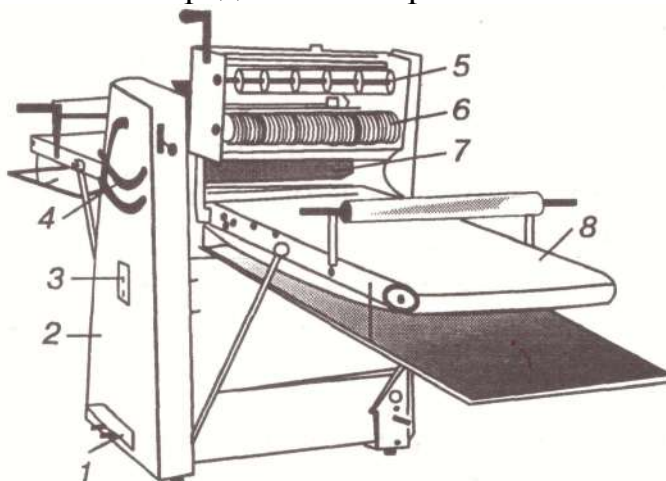
Рис. 52 – Машина МНРТ-130/600 для розкочування тіста:
