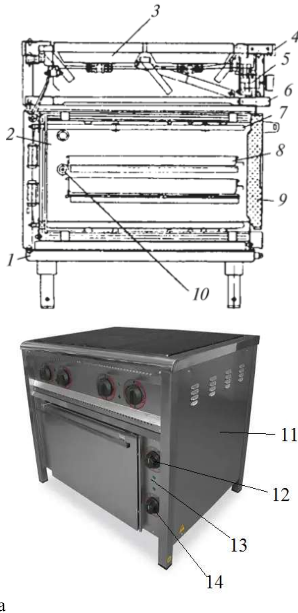
Рис. 84 – Плита електрична секційна модульна ПЕСМ-4Ш:
