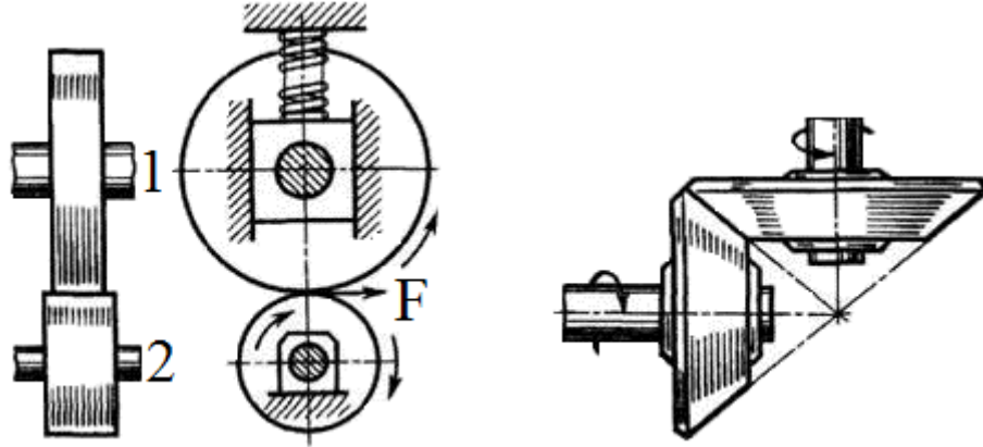
Рис. 23 – Фрикційні передачі
