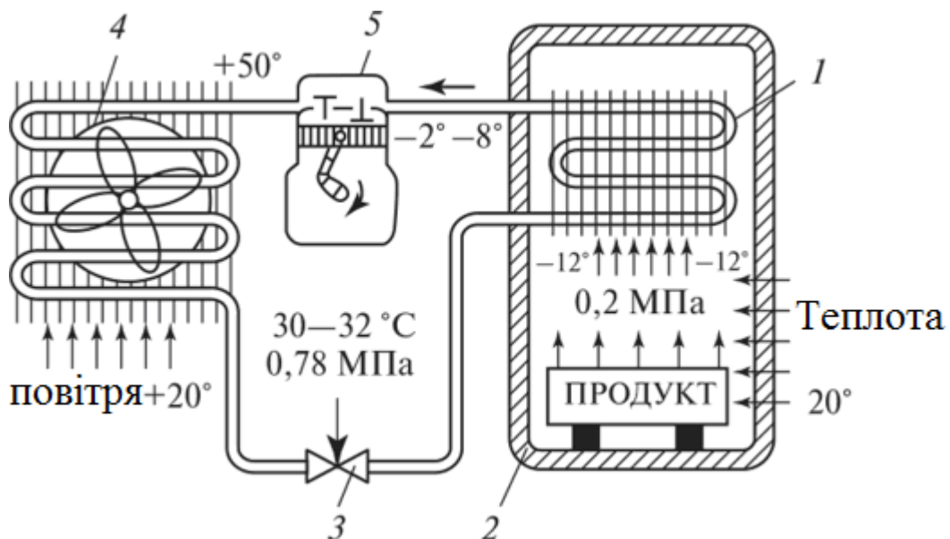
Рис. 108 – Схема компресійної холодильної машини:
