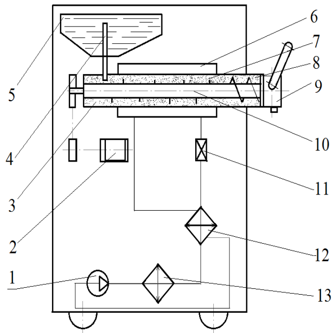
Рис. 130 – Принципова схема фризера:
