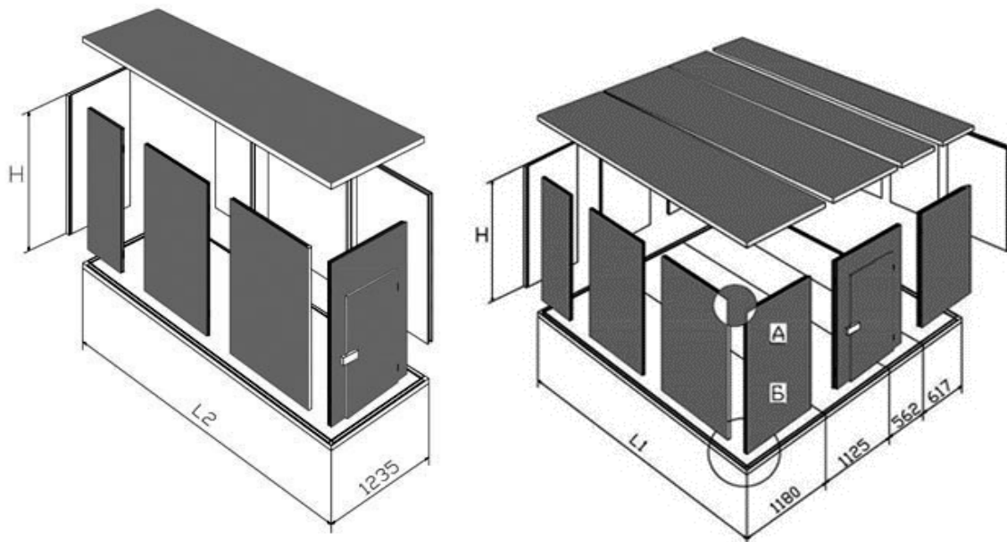
Рис. 114 – Збірні середньо- та низькотемпературні холодильні камери з товщиною ізоляції 80 мм
