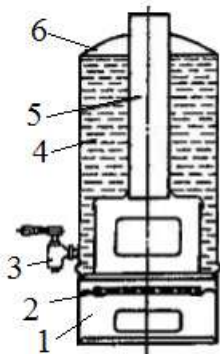
Рис. 94 – Кип'ятильник наливний принципова
