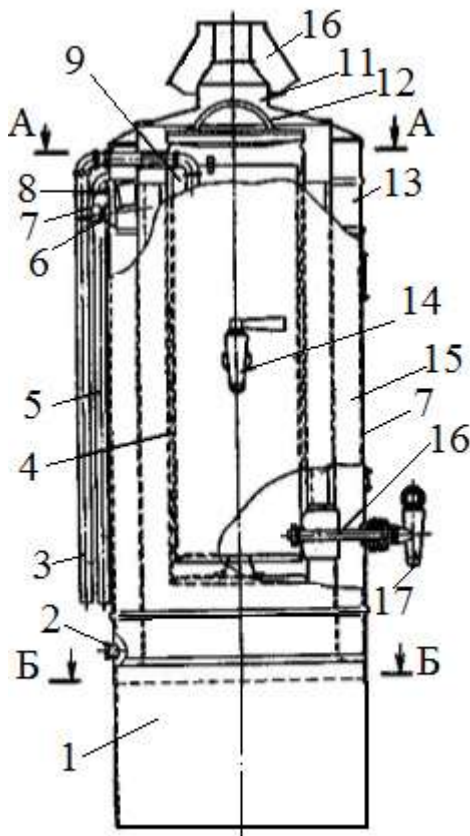
Рис. 97 – Кип'ятильник безперервної дії газовий принципова схема:
