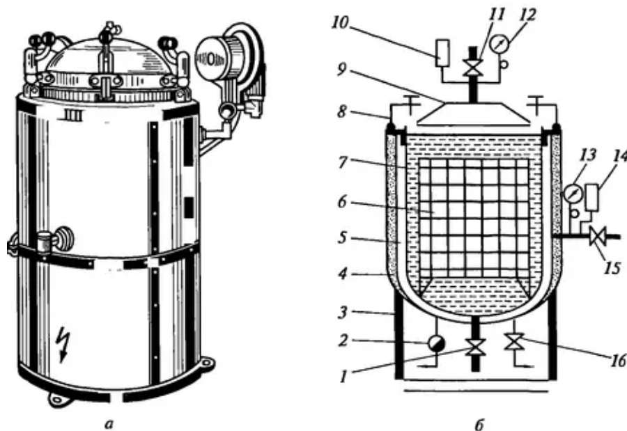
Рис. 61 – Паровий автоклав:
