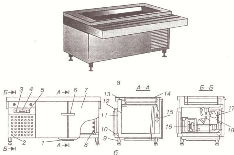
Рис. 119 – Холодильний прилавок-вітрина ЛС-2М:
