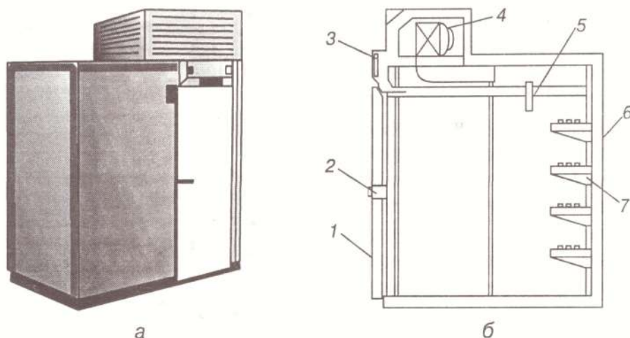
Рис. 112 – Камера холодильна КХС-1-8,0:
