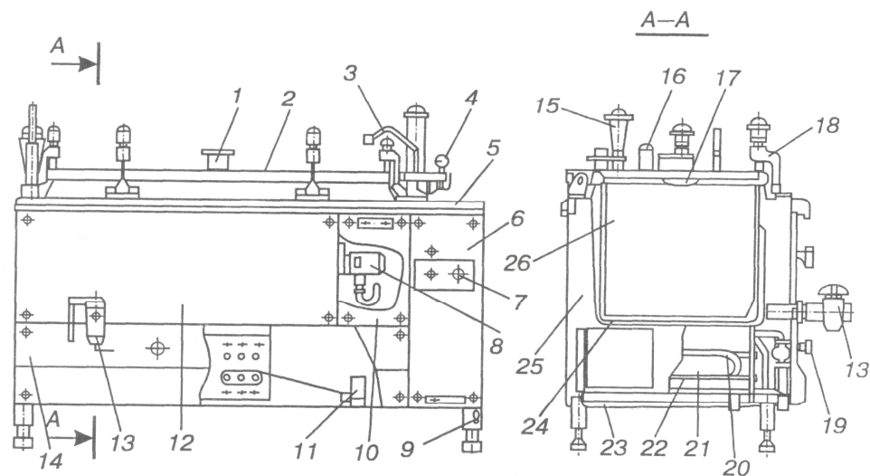
Рис. 59 – Котел харчоварильний KE-100М (KE-160М, KE-250):
