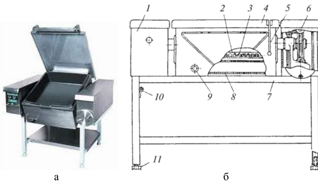
Рис. 69 – Сковорода електрична секційна модульна СЕСМ-0,2: а – загальний вигляд; б – у розрізі
