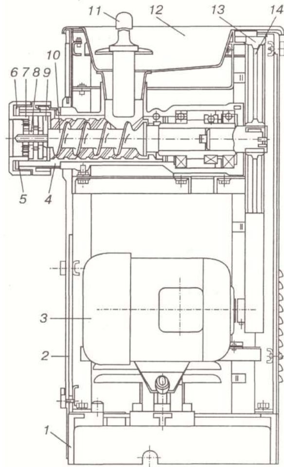
Рис. 30 – Схема м'ясорубка МЗМ-105М:
