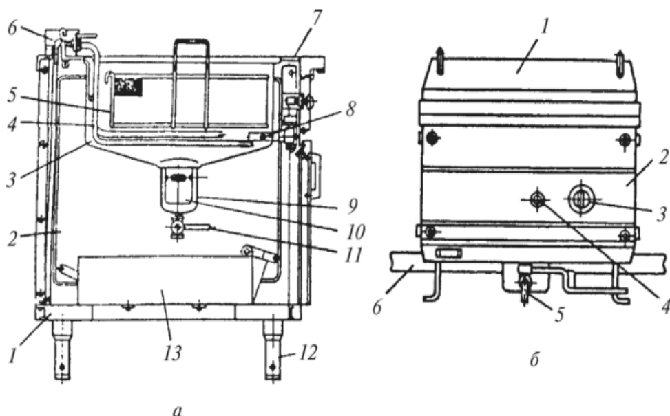
Рис. 75 – Фритюрниці електричні принципова схема: а – ФЕСМ-20 (у розрізі); б – ФЕ-20
