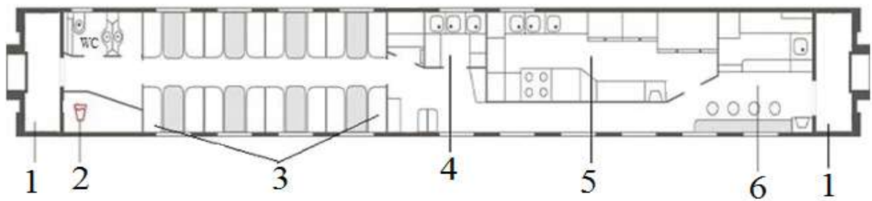
Рис. 8 – Схема вагона-ресторану:
