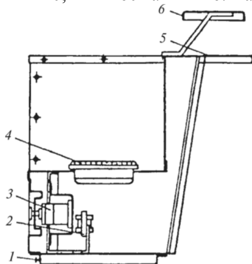
Рис. 100 – Марміт для перших страв принципова схема:
