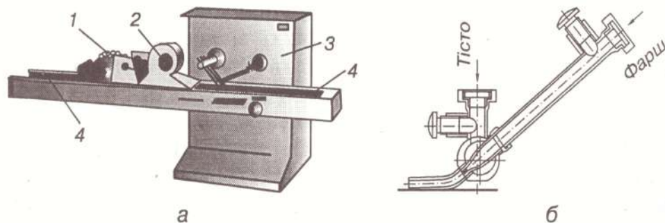
Рис. 50 – Машина ВМП для формування вареників та пельменів:
