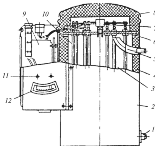
Рис. 98 – Водонагрівач НЕ-1Б:
