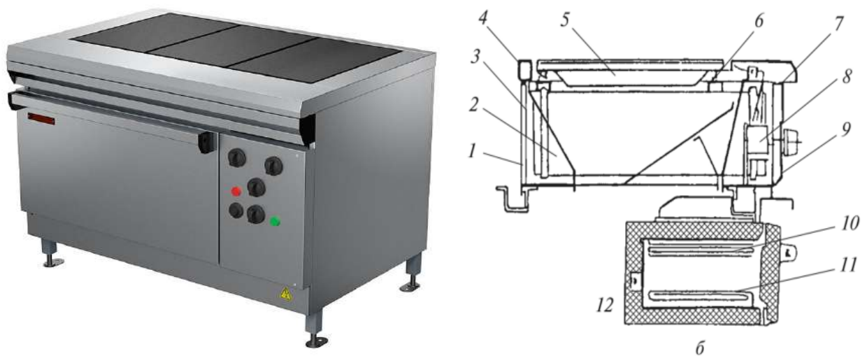
Рис. 87 – Плита електрична з жаровою шафою ПЕ-0,51 Ш:
