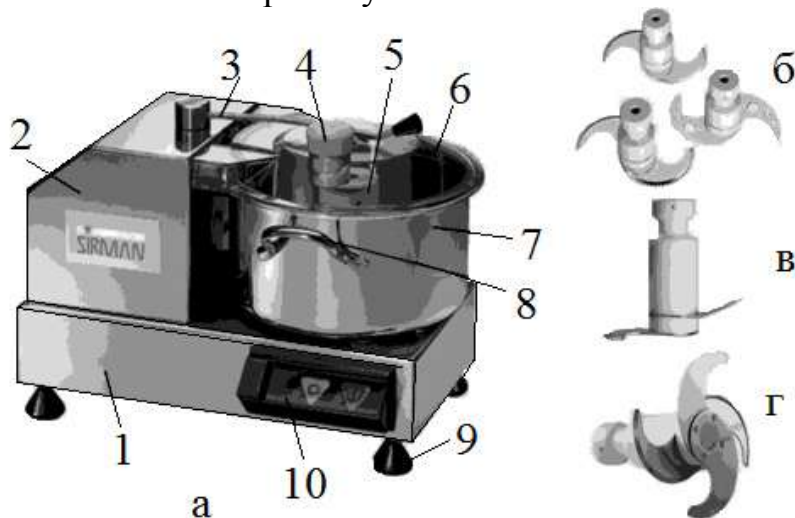
Рис. 36 – Кутер С4W:
