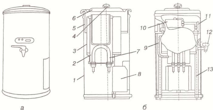
Рис. 96 – Кип'ятильник КБЕ-25МІ (КБЕ-50МІ):
