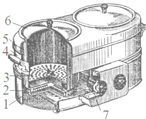
Рис. 66 – Сосисковарка принципова схема:
