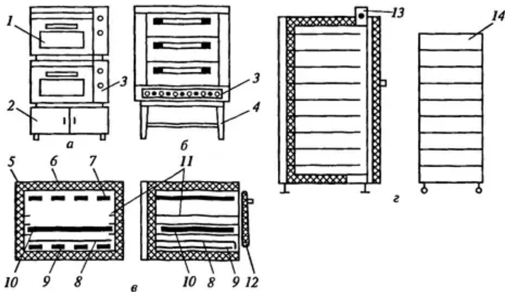
Рис. 77 – Принципова схема жарових та кондитерських шаф із природньою конвекцією:
