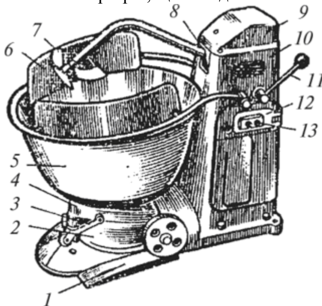
Рис. 49 – Тістомісильна машина ТММ-1М
