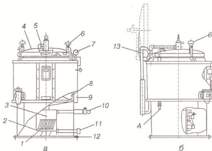
Рис. 57 – Принципова схема котла для перших страв КХЕ-160-ІМ-10:
