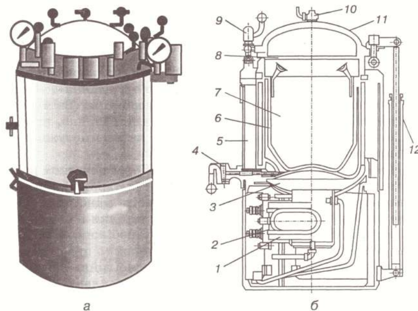
Рис. 62 – Автоклав АЕ-1:
