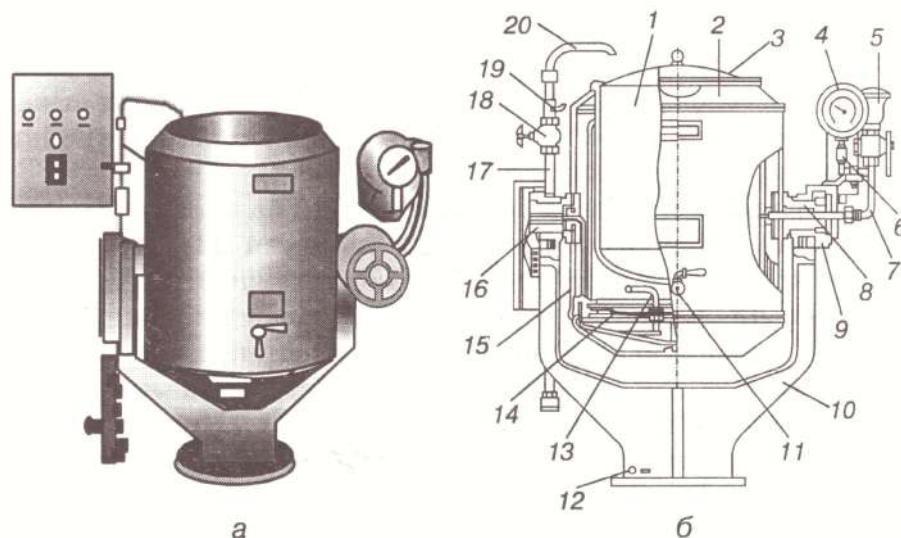
Рис. 58 – Котел харчоварильний електричний КХЕ-60:
