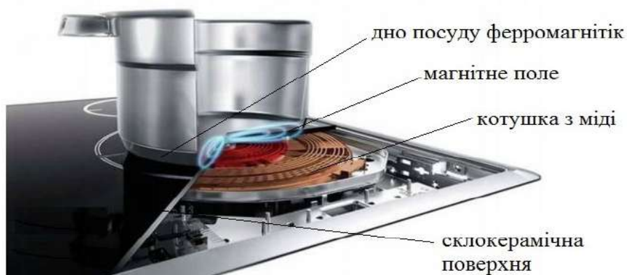
Рис. 90 – Будова індукційної плити
