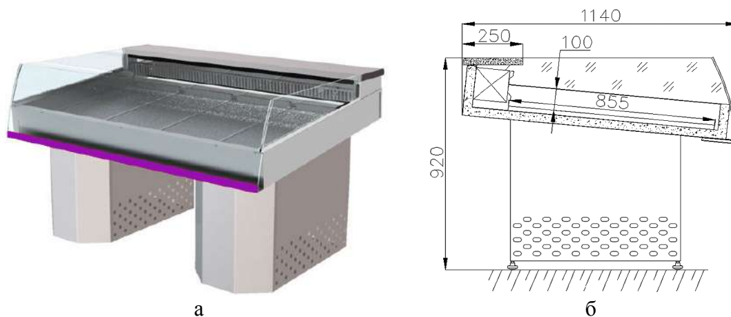
Рис. 120 – Холодильная витрина ВУ 17: а – загальний вид; б – габаритні розміри
