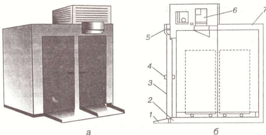
Рис. 113 – Камера холодильна КХС-1-8,ОК:
