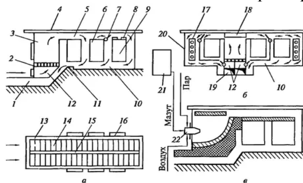
Рис. 93 – Вогневі плити:
