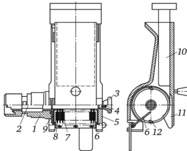
Рис. 34 – Схема механізму для нарізання м'яса на бефстроганів:
