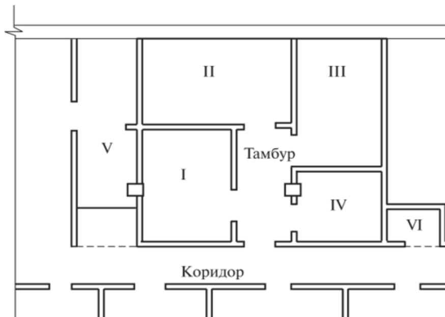
Рис. 110 – Розташування стаціонарних холодильних камер:
