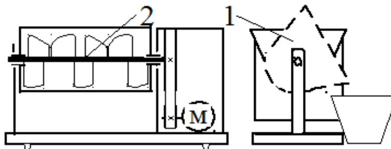
Рис. 32 – Принципова схема фаршемісу
