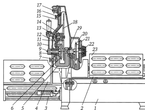
Рис. 40 – Схема машини для нарізання хлібу МРХ-200:
