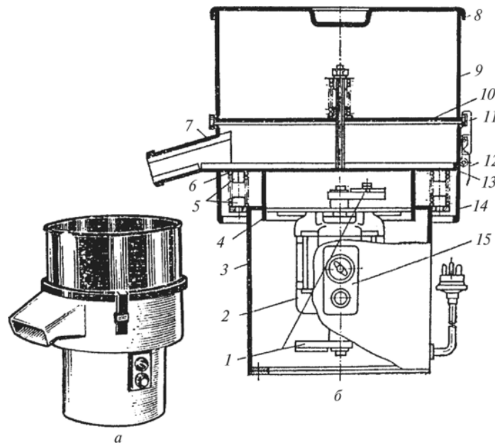
Рис. 48 – Малогабаритний просіювач борошна вібраційний МПМВ-300: а – загальний вид; б – у розрізі
