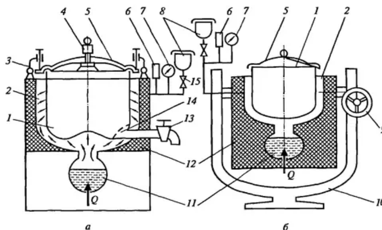
Рис. 55 – Принципові схеми котлів з непрямым обігрівом стінки варильного посуду:
