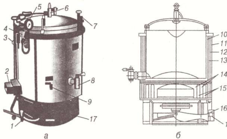
Рис. 60 – Котел харчоварильний газовий КХГ-250:
