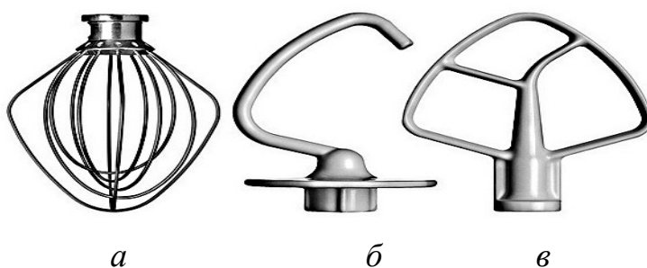
Рис. 53 – Насадки для збивальної машини:
