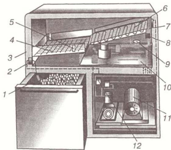
Рис. 129 – Льодогенератор, принципова схема:
