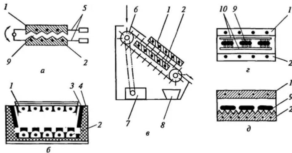
Рис. 70 – Принципові схеми сковорід із двостороннім обігрівом виробів:
