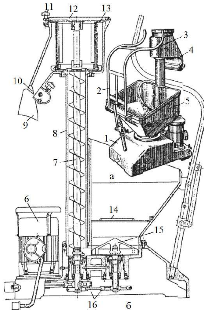
Рис. 47 – Машина для просіювання МПБ-800
