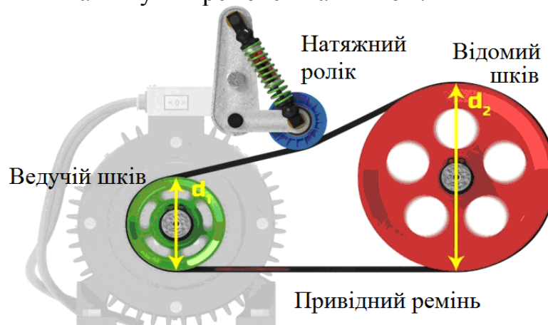
Рис. 22 – Загальна схема устаткування ремінної передачі
