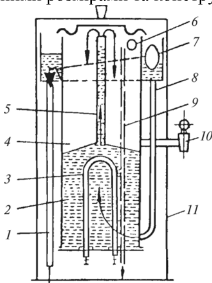
Рис. 95 – Принципова схема електрокип'ятильника безперервної дії:
