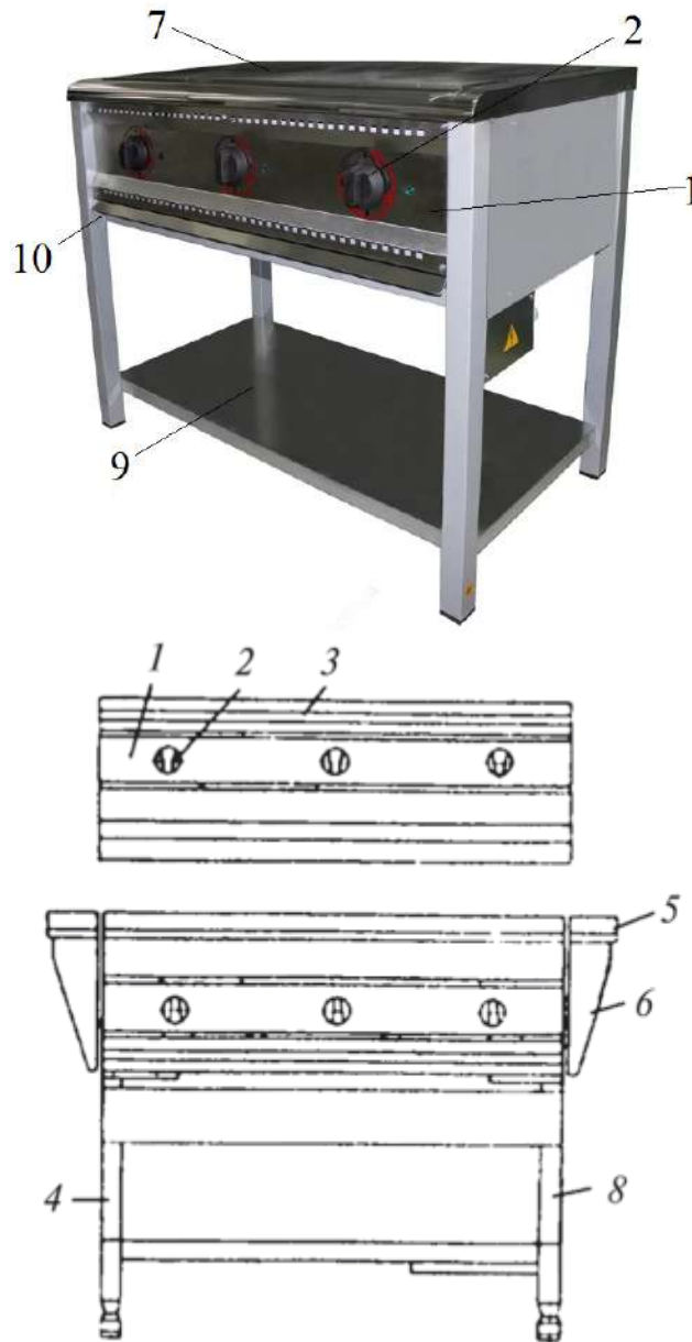
Рис. 85 – Плита електрична : а – ПЕ-0,51(зовнішній вигляд) та ПЕ-0,51-01 (розріз)
