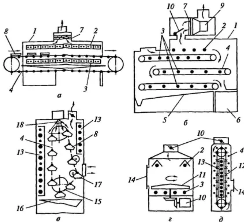
Рис. 83 – Принципові схеми ІЧ-апаратів безперервної дії:
