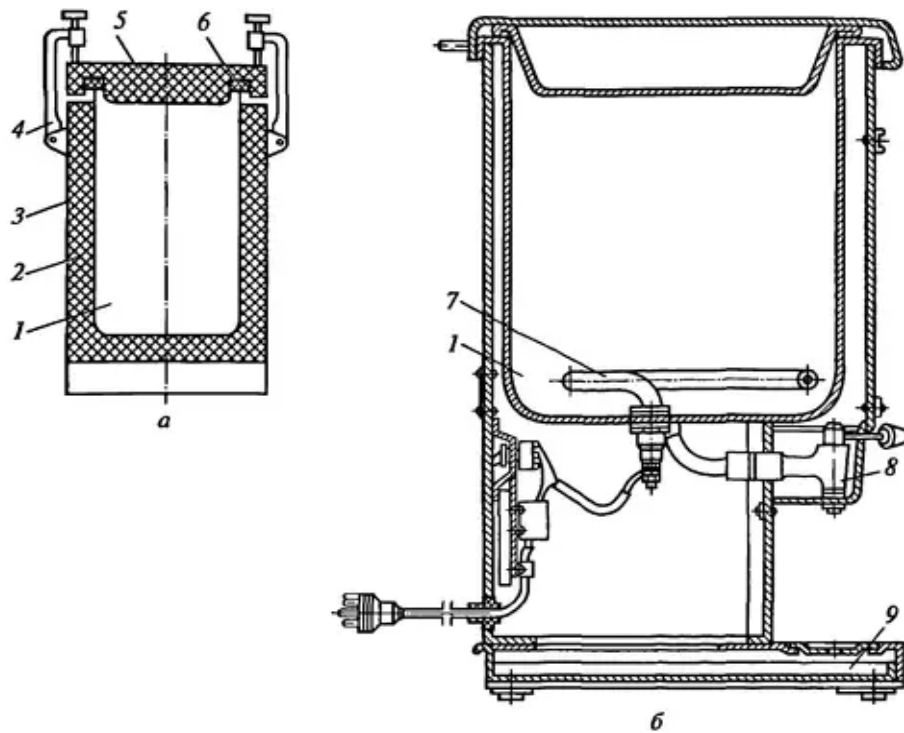
Рис. 106 – Принципова схема термостатів:
