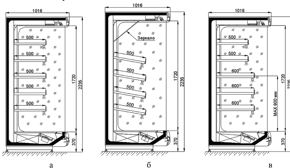
Рис. 126 – Габаритні розміри гірок «Корделія»:
