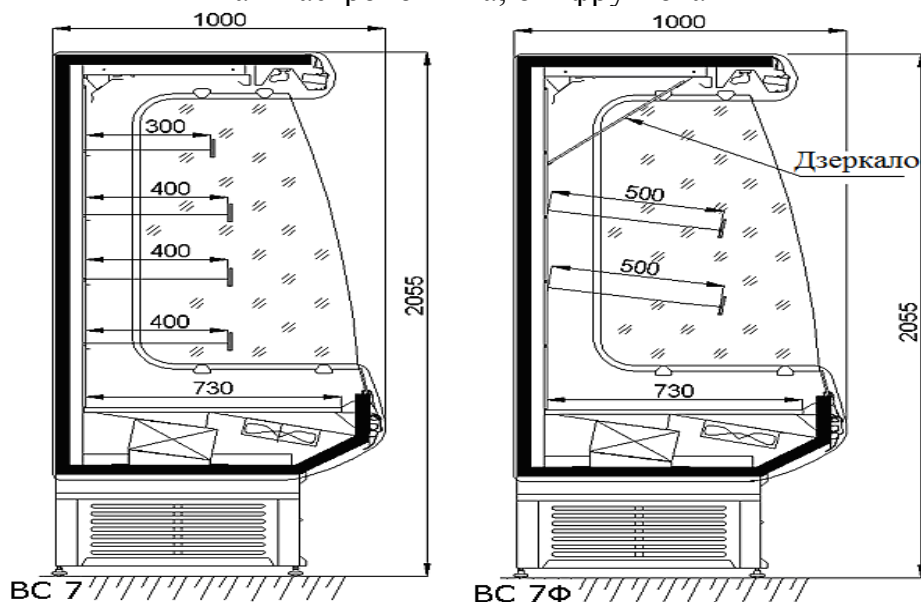
Рис. 124 – Габаритні розміри гірки «Віола»
