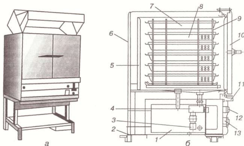
Рис. 64 – Апарат пароварильний АПЕ-0,23АМ-01 (а – загальний вигляд), АПЕ-0,23АМ (б – розріз):
