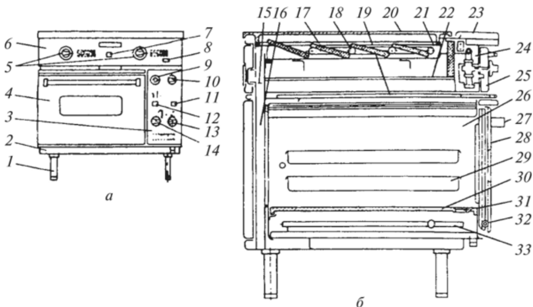
Рис. 91 – Плита газова ПСГМ-2Ш:
