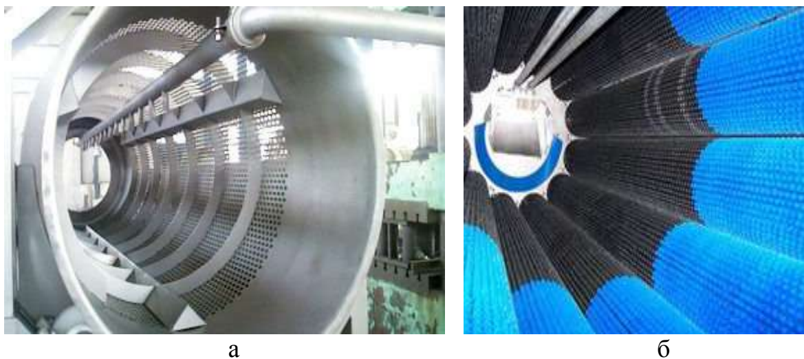
Рис. 25 – Мийна машина барабанного типу: а – барабан без щіток; б – барабан із щітками
