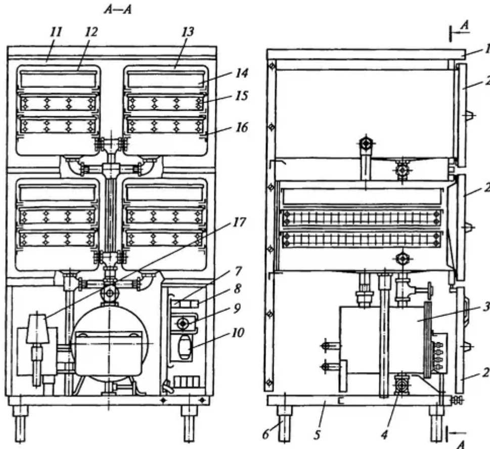
Рис. 63 – Паровий варильний апарат АПЕСМ-2:
