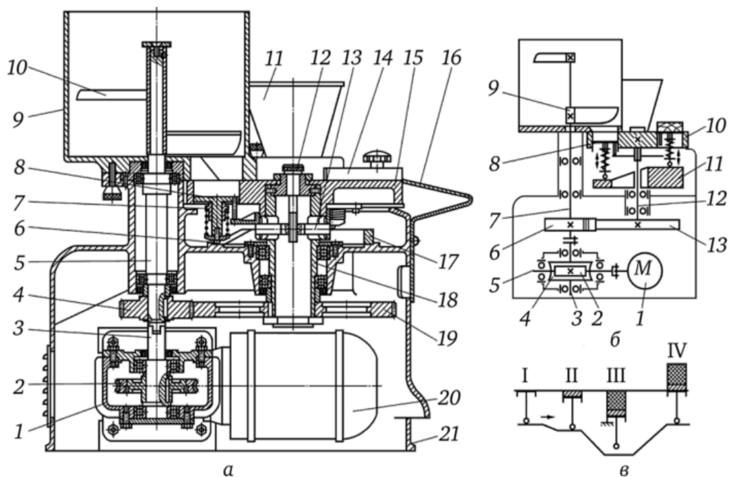
Рис. 37 – Схема машини для формування котлет МФК-2240:
