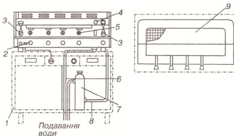
Рис. 65 – Принципова схема електричної кавоварки:
