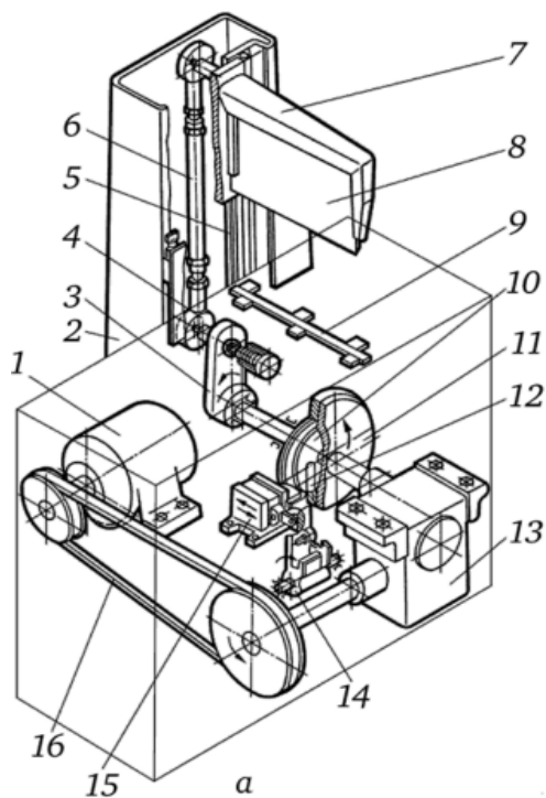
Рис. 46 – Машина для нарізання заморожених продуктів:
