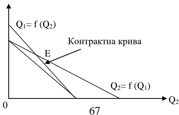
Рисунок 5.5 – Модель Курно
