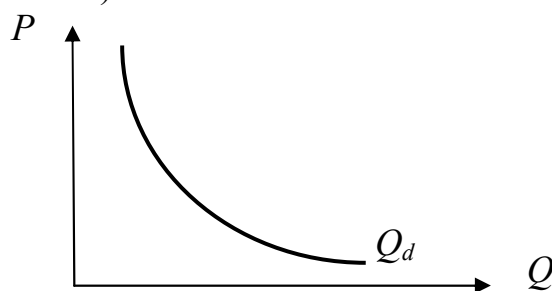
Рис. 4.1. Крива попиту
