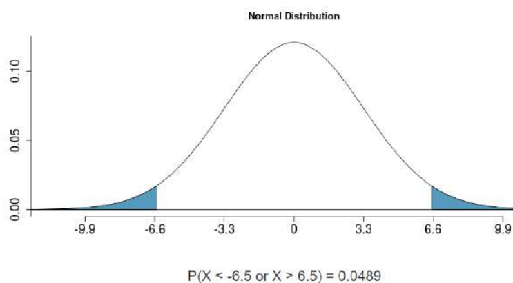
Рис. 3.2. Нормальний розподіл
