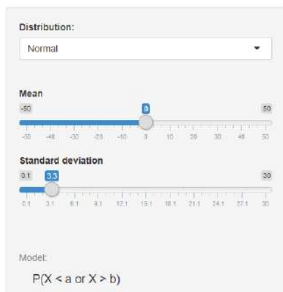
Рис. 3.2. Нормальний розподіл
