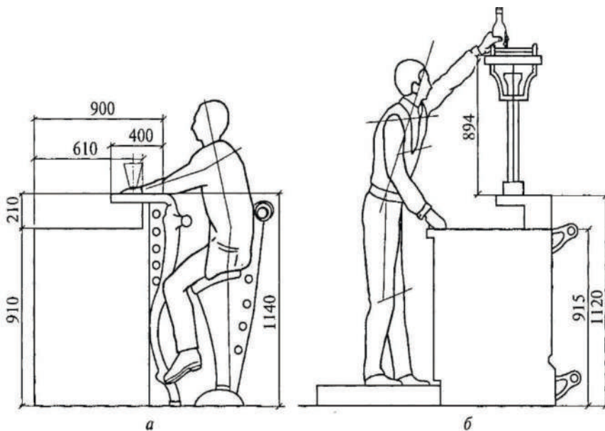
Мал. 2.2.1. Стандартні розміри барної стойки:
