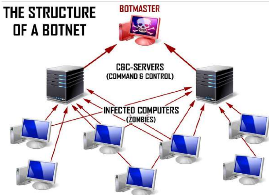
Рис. 6.7. Структура бот-мережі
